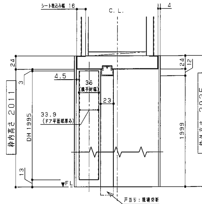
縦詳細図
