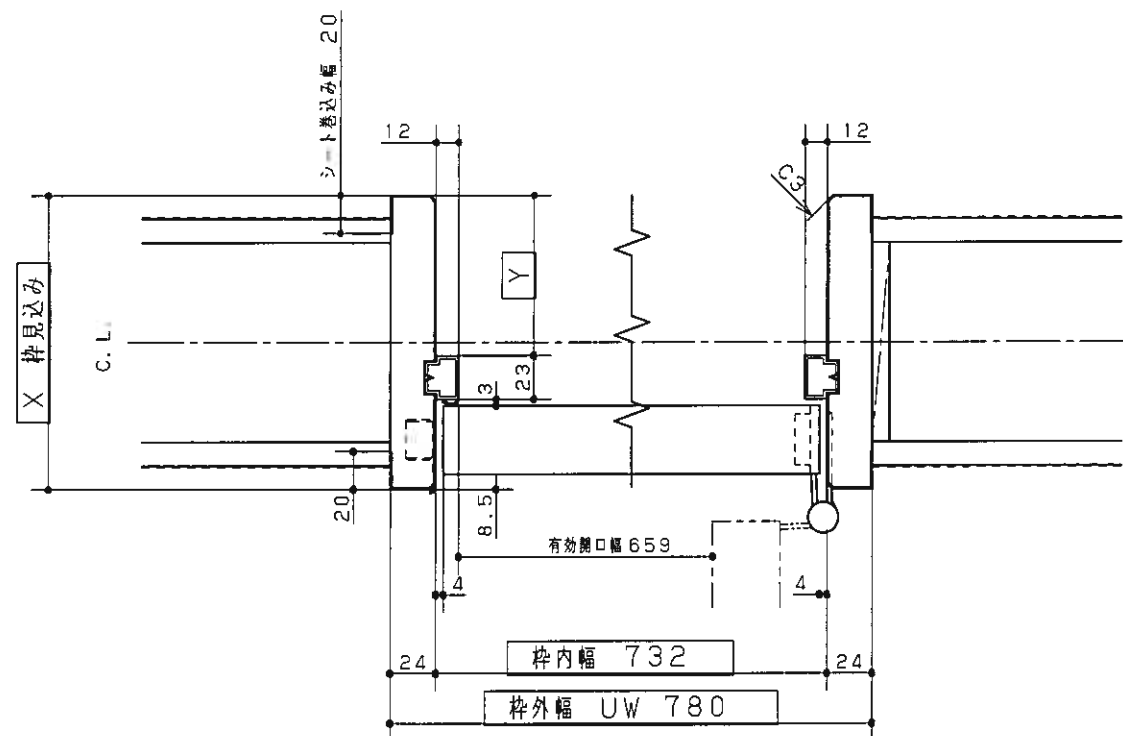
横詳細図
